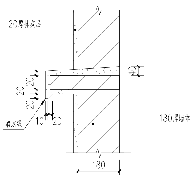
窗台抹灰大样图
